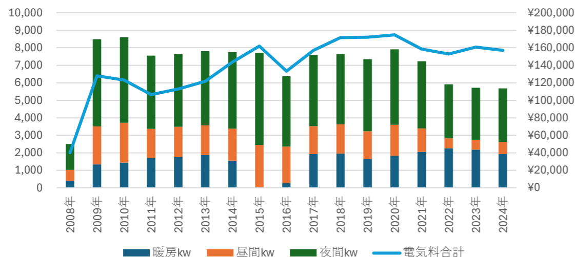
使用電力と光熱費合計
